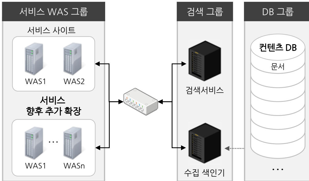
<하드웨어 구성도>
